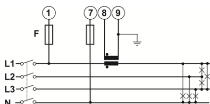
Fig. 7 AV5, AV6 balanced load
