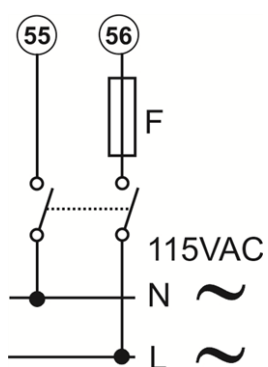
Fig. 23 D option. F = 250\text{ V}, 100\text{ mA}
