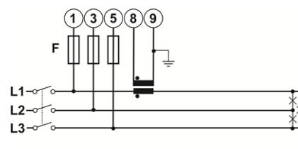
Fig. 13 AV5, AV6 balanced load
