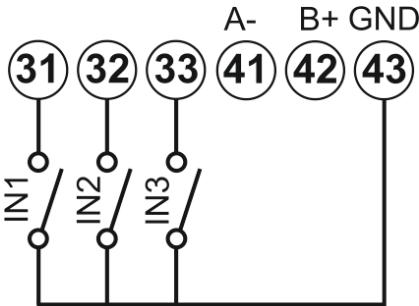
Fig. 28 Digital inputs
