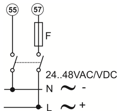
Fig. 24 L option. F = 250\text{ V}, 200\text{ mA}
